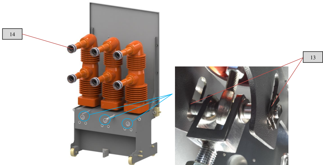
Рис. 16 Места смазки согласно табл. 12
