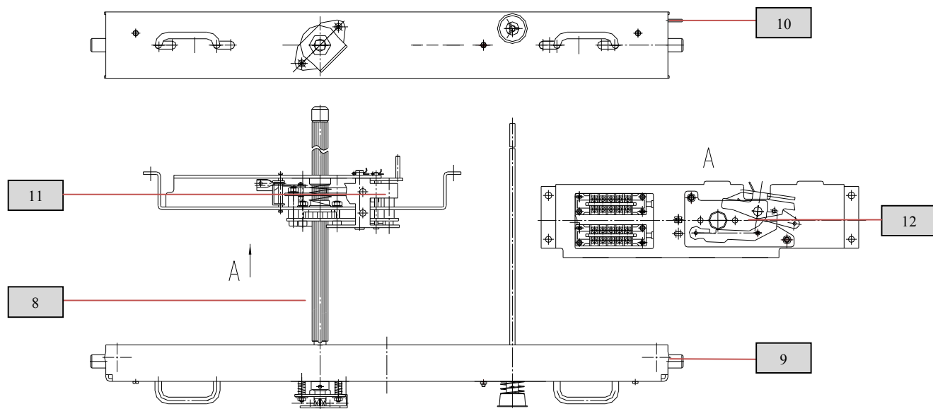
Рис. 15 Места смазки подвижных узлов тележки аппаратной согласно табл. 12
