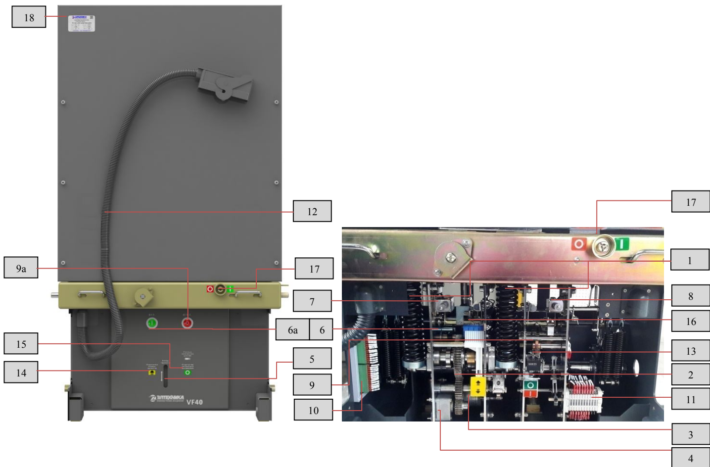
Рис. 3 Привод выключателя
