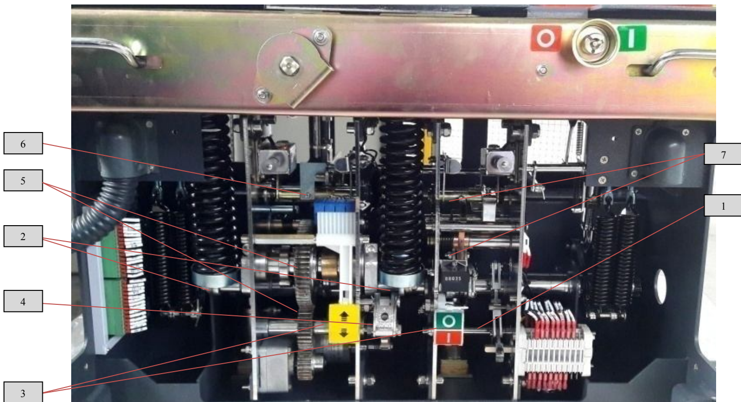
Рис. 14 Места смазки подвижных узлов в приводе выключателя: обозначения см. табл. 12
