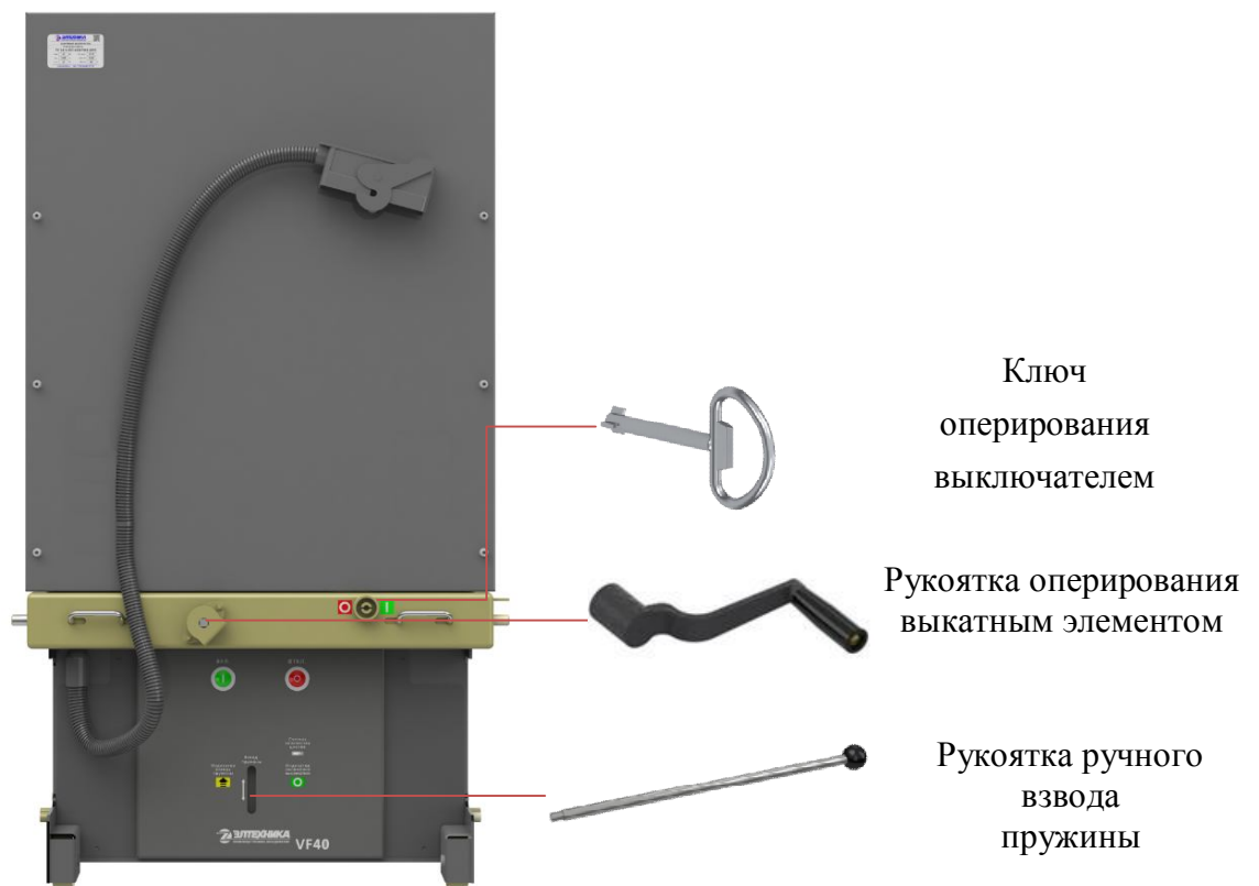
Рис. 9 Рукоятки
