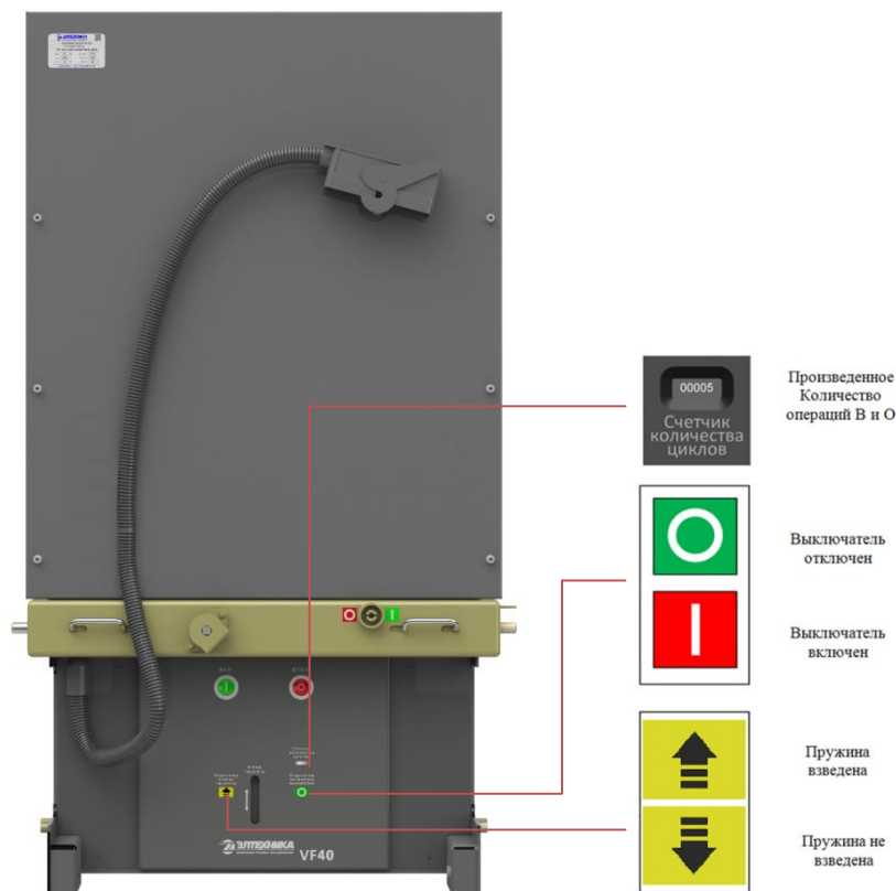
Рис. 4 Индикаторы на лицевой панели выключателя
