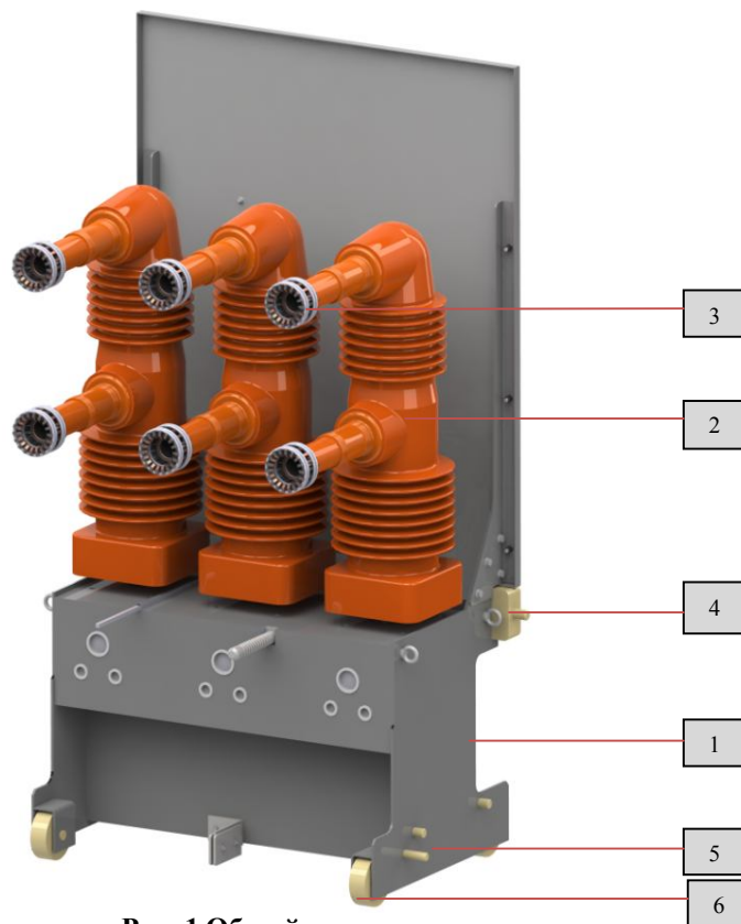
Рис. 1 Общий вид выключателя
