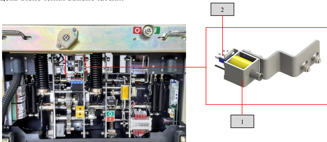
Рис. 6 Электромагнитная блокировка включения
