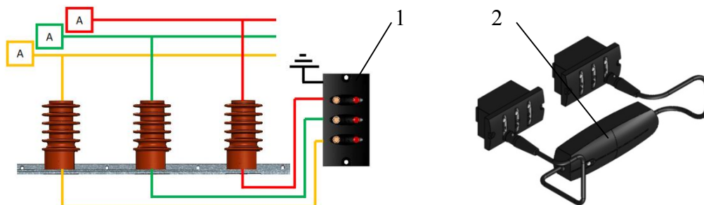
Рис. 10. Схема соединения блока индикации напряжения 1 – блок индикации напряжения; 2 – устройство для фазировки
