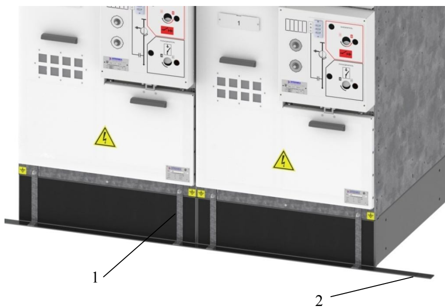
Рис. 16б. Пример монтажа контура заземления КСО: 1 – уголок из оцинкованной стали 3x25; 2 – стальная полоса 4x40
