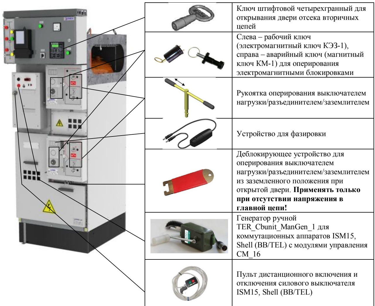
Рис. 5. Принадлежности КСО
