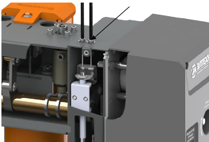
Рис. 5.1 Установка тросика в выключателе VF12
