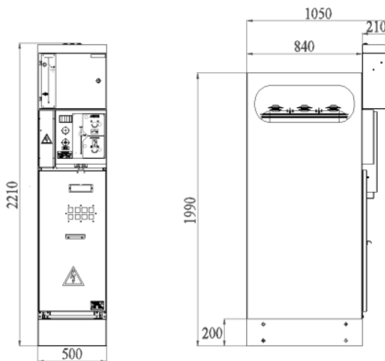
Рис. 2.5. Габаритные размеры КСО габарит 1 и 2 с шириной корпуса 500 мм
