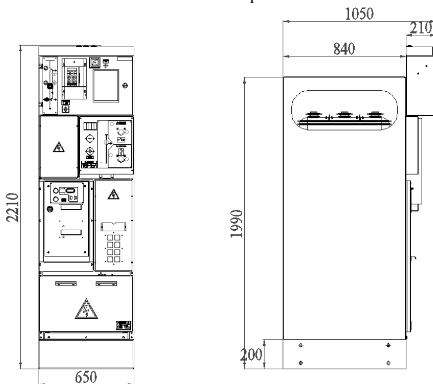
Рис. 2.3. Габаритные размеры КСО габарит 1 и 2 с шириной корпуса 650 мм
