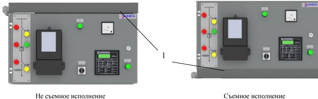
Рис. 2а. Отсек вторичных цепей 1 – съемная планка кабельного канала
