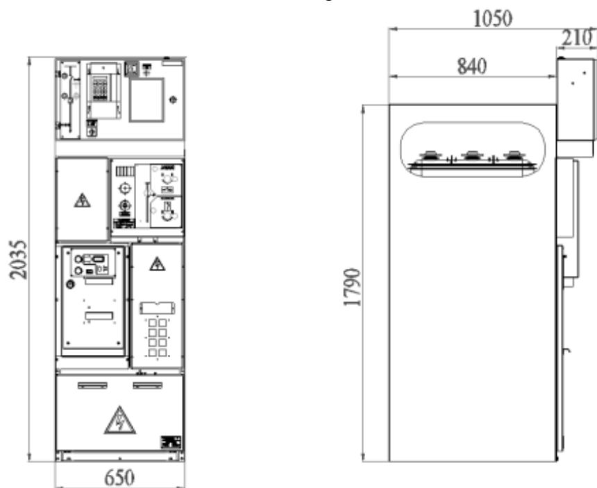
Рис. 2.4. Габаритные размеры КСО габарит 3 и 4 с шириной корпуса 650 мм
