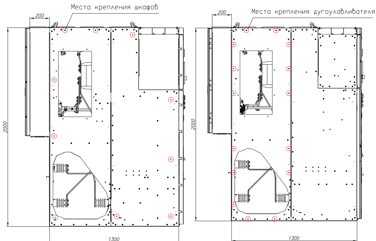
Рис. 22 Места скрепления соседних шкафов КРУ
