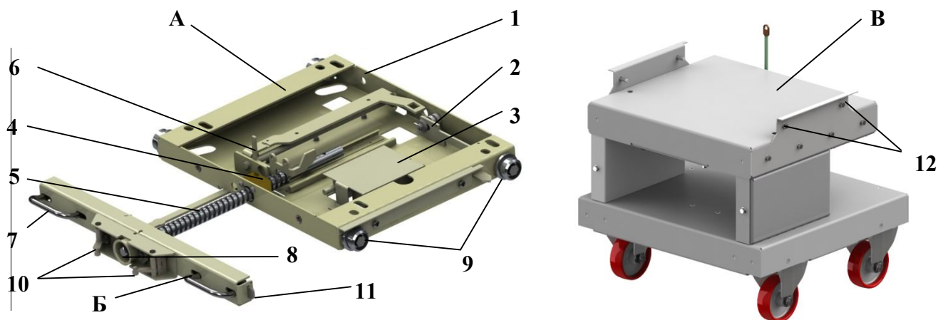
Рис. 8 Тележка аппаратная:
