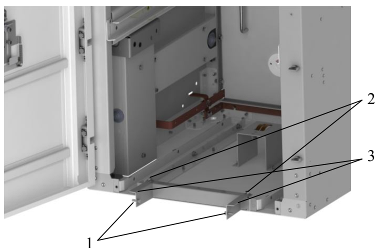
Рис. 31 Монтаж выкатных элементов
