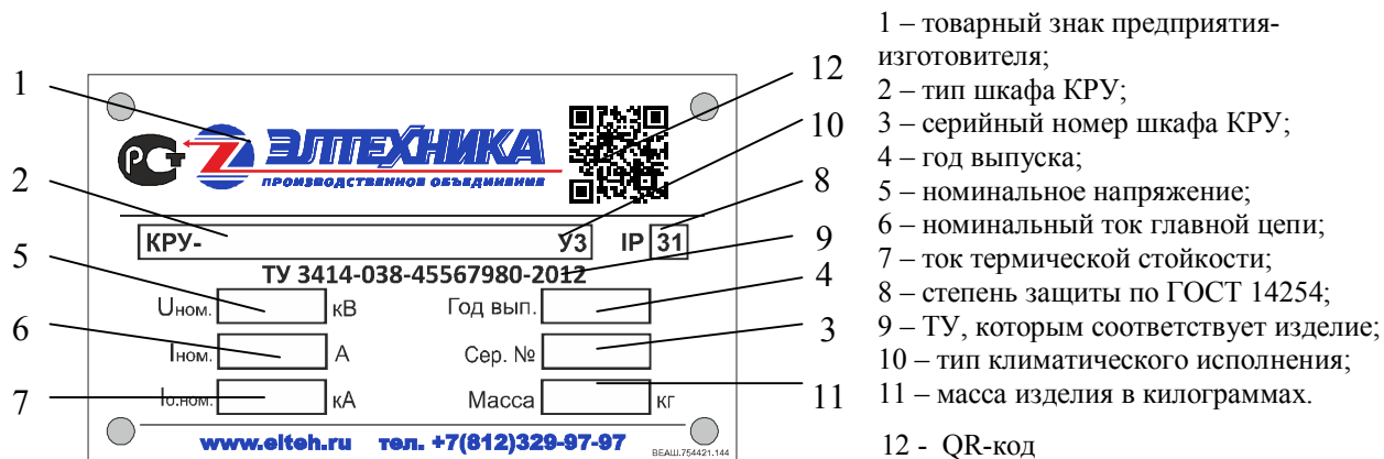
Рис. 5 Маркировочная табличка
