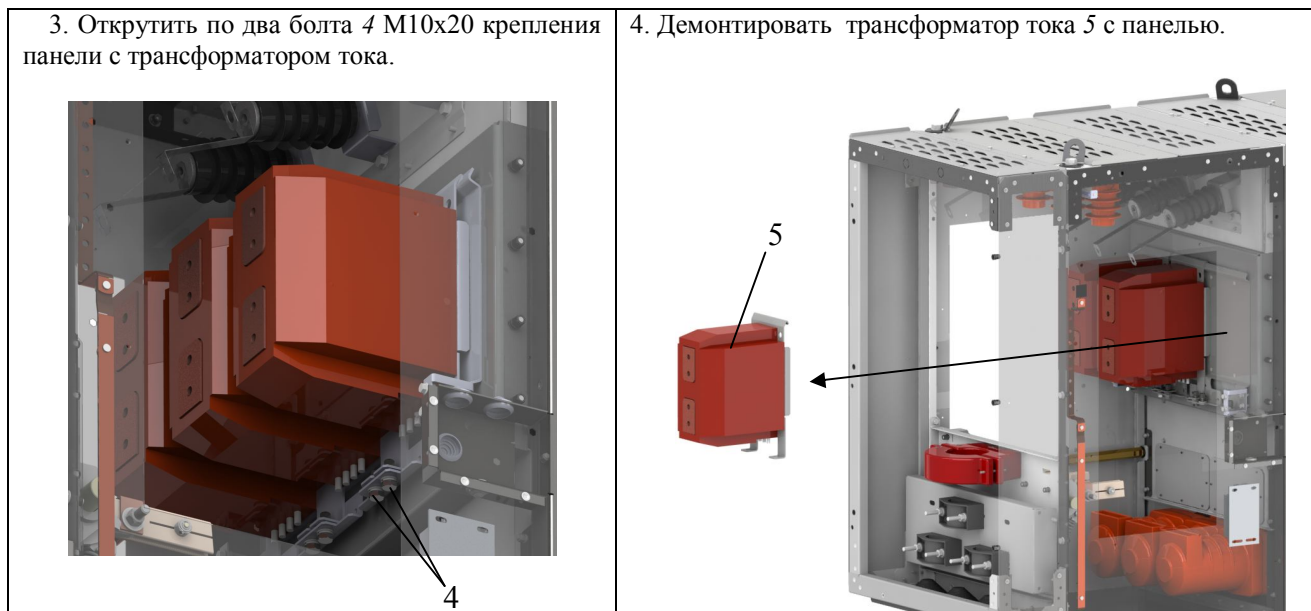
Рис. 37. Порядок демонтажа измерительных трансформаторов тока
