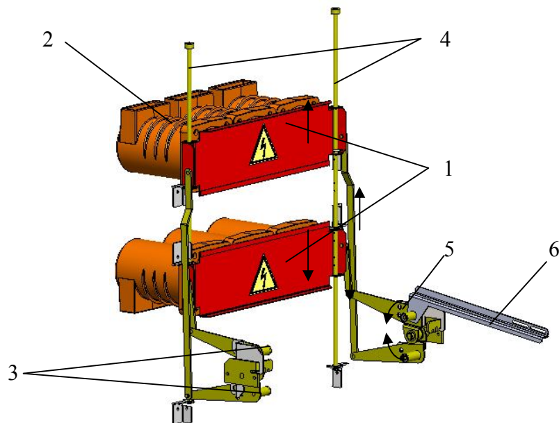
Рис. 10 Шторочный механизм
