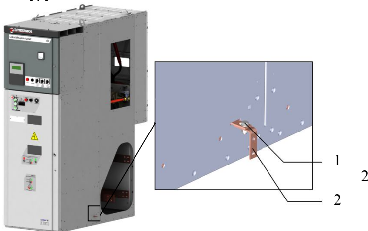
Рис. 24 Сборка системы заземления секции шкафа КРУ 1 – болтовое соединение М8; 2 – шина заземления соседнего шкафа КРУ
