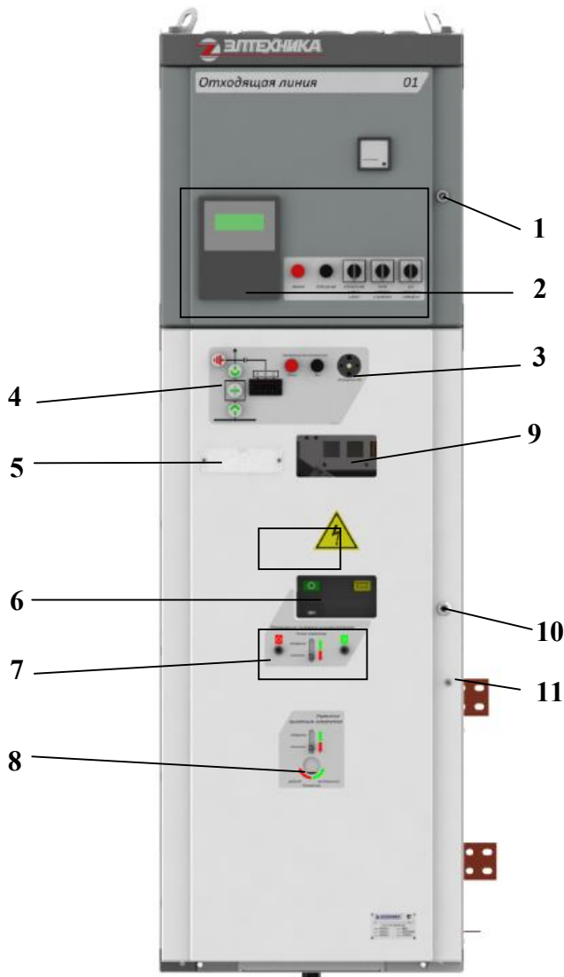
Рис. 2 Лицевая сторона шкафа КРУ
