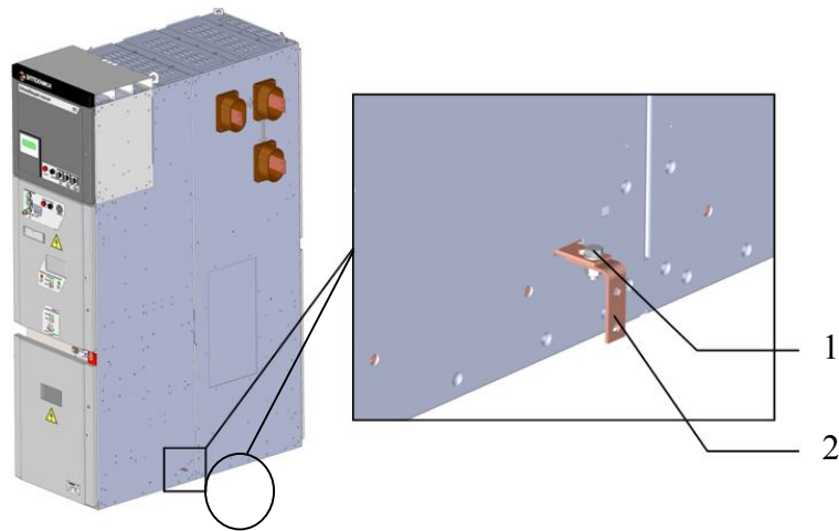
Рис. 23 Сборка системы заземления секции шкафов КРУ 1 – болтовое соединение М8; 2 – шина заземления соседнего шкафа КРУ
