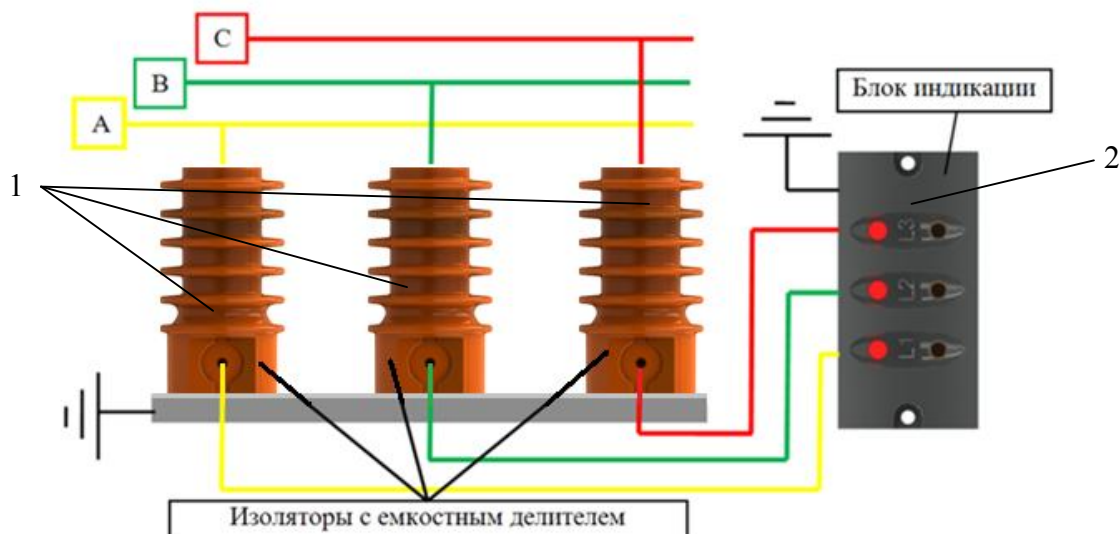
Рис. 12 Схема соединения блока индикации напряжения
