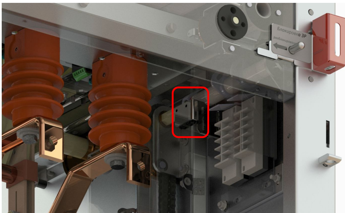
Рис. 4.1 Внешний вид концевых переключателей моторизованного привода заземлителя.
