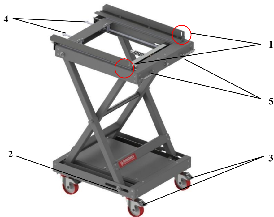
Рис. 9 Сервисная тележка:
