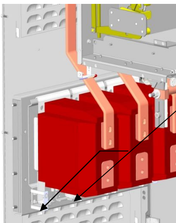
Рис. 27 Порядок демонтажа измерительных трансформаторов тока
