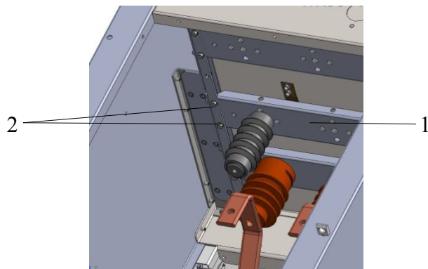
Рис. 26 Планка с ОПН
