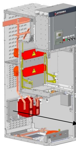
Рис. 27 Порядок демонтажа измерительных трансформаторов тока
