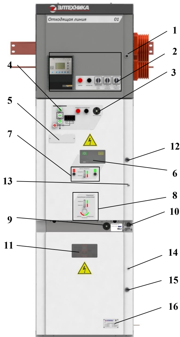
Рис. 2 Лицевая панель КРУ
