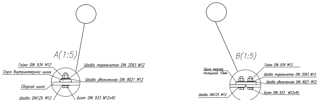
Рис. 25 Монтаж сборных шин А – крепление шины 10x40 отходящей линии; В – соединение сборных шин
