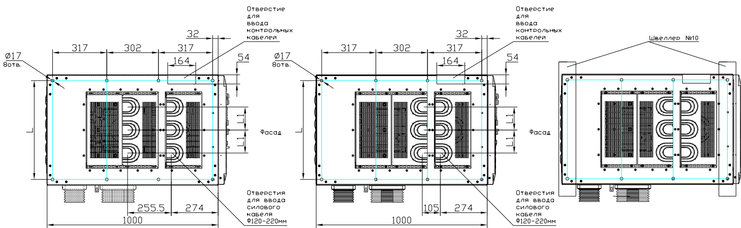
Рис. 2.2 Установочные размеры шкафов КРУ
