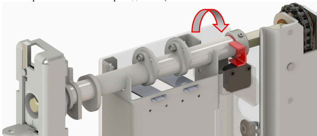
Рис. 4.3 Крайнее положение привода вала (заземлитель в положении «Заземлен»).
