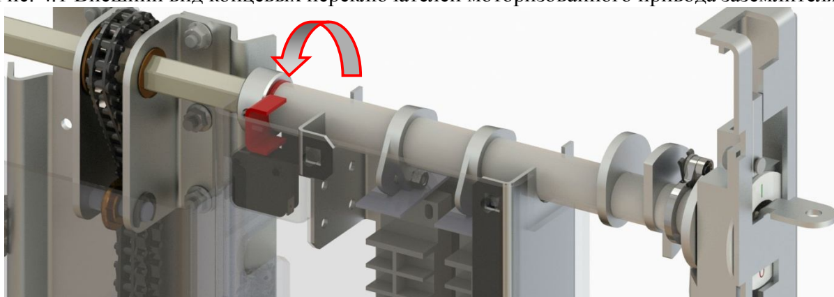
Рис. 4.2 Крайнее положение привода вала (заземлитель в положении «Отключен»).
