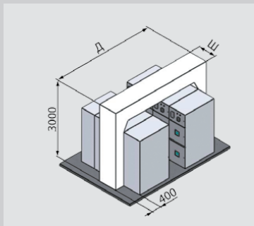
Шинный мост двухсекционного РУ
