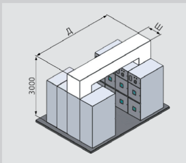
Шинный мост односекционного РУ
