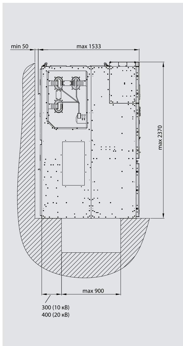
ВИД СБОКУ
